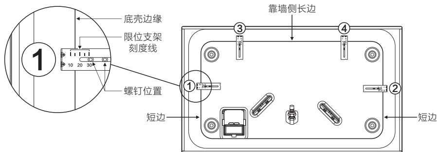
图（11）限位支架安装位置示意图
