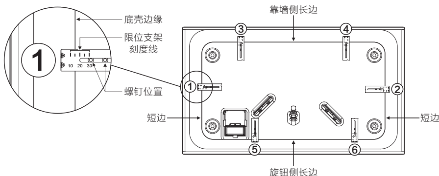
(图12) 限位支架安装位置示意图
