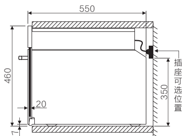
安装侧视图
