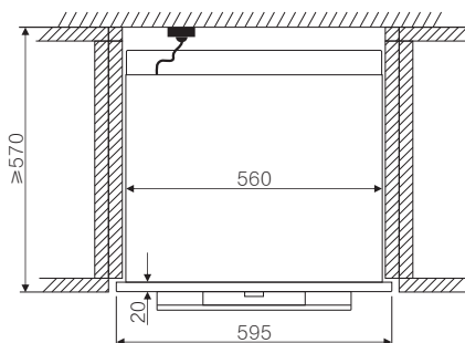
安装俯视图
