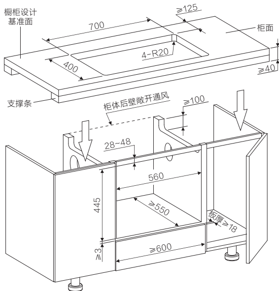
方案二：增加夹板安装柜体设计图
