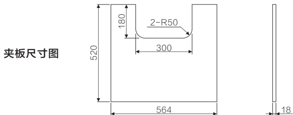
方案二：增加夹板安装柜体设计图
