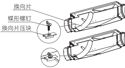
图（3）左侧出风换向片安装示意图
